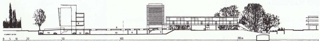
ΤΟΜΗ Β-Β ΣΥΝΟΛΙΚΗΣ ΠΡΟΤΑΣΗΣ
