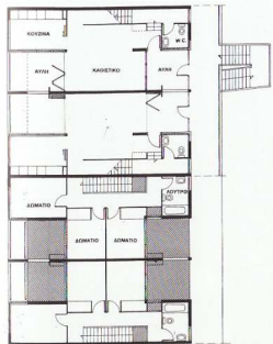
ΔΙΩΡΟΦΗ ΚΑΤΟΙΚΙΑ: ΙΣΟΓΕΙΟ+ΟΡΟΦΟΣ
