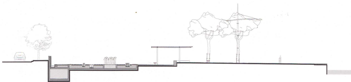
Κήπος του Νερού. Τομή Water Garden. Section
