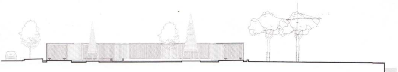
Κήπος των Ρόδων. Τομή Rodes Garden. Section
